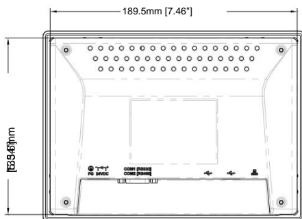
背视图
