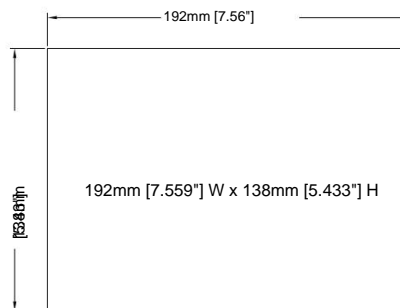
开孔尺寸图
